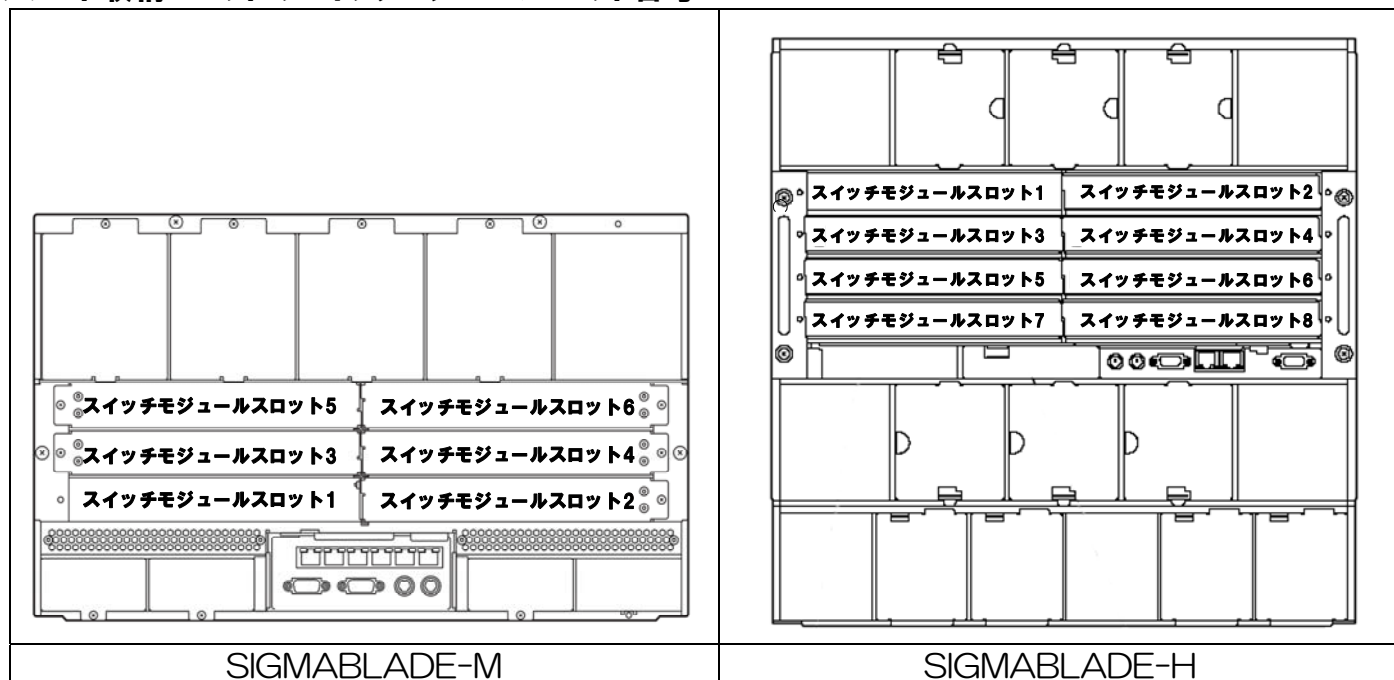
ブレード収納ユニット背面
